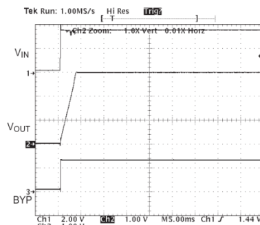
Fig. 17: Fast V_{IN} = 1000µF Output Load
