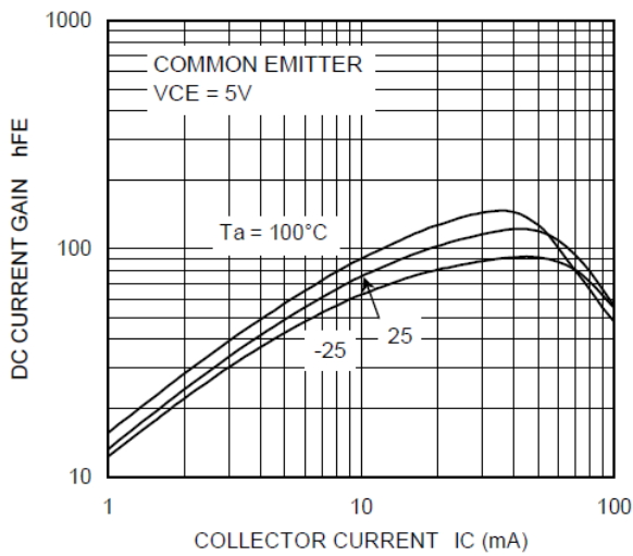
Fig. 10.13 RN1416 h_{FE}-I_C
