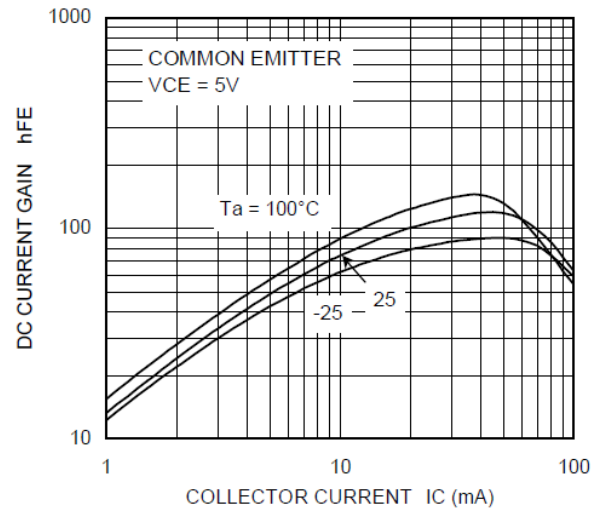
Fig. 10.12 RN1415 h_{FE}-I_C
