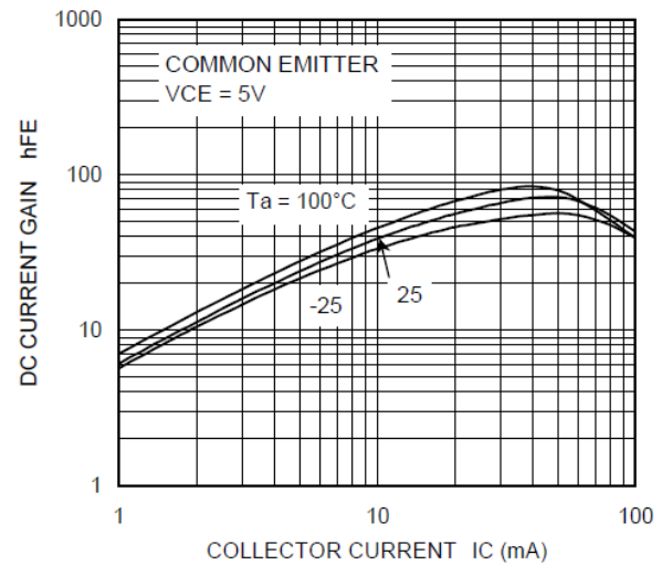
Fig. 10.14 RN1417 h_{FE}-I_C
