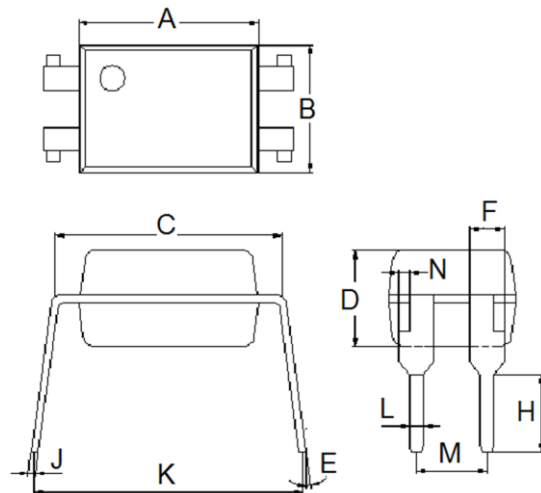
DIP-4
