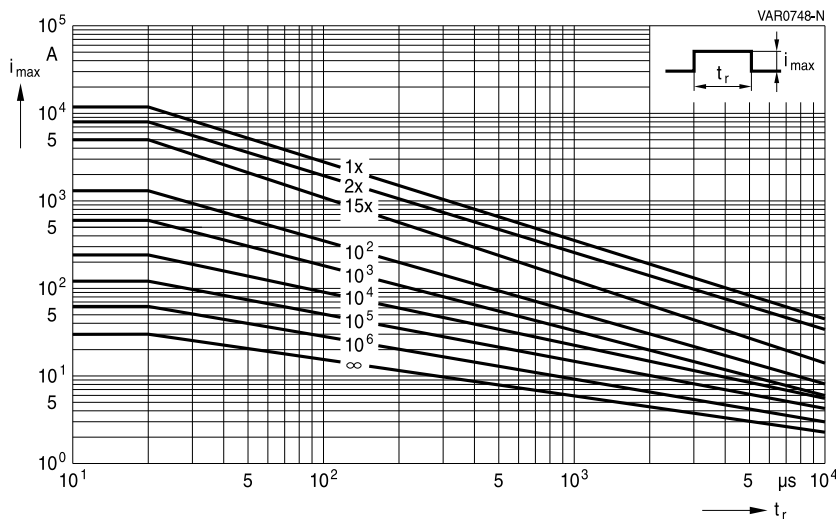
SIOV-SNF20K130 ... K320E3S5K1
