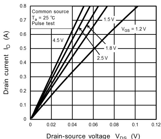
Fig. 7.1 I_D - V_{DS}
