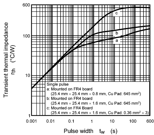
Fig. 7.11 r_{th} - t_w
