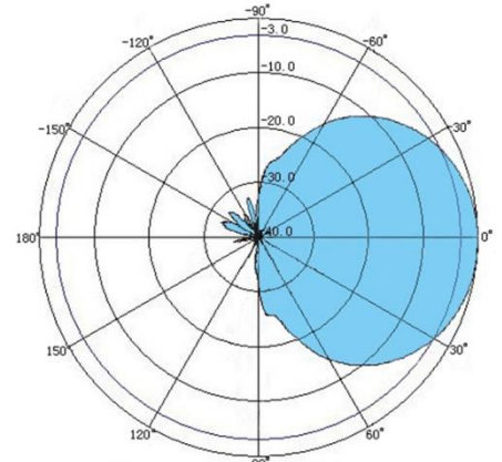
1710-3800MHz
