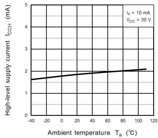
Fig. 13.2.6 I_{CCH} - T_a
