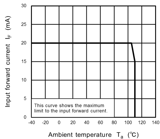
Fig. 13.2.2 I_F - T_a
