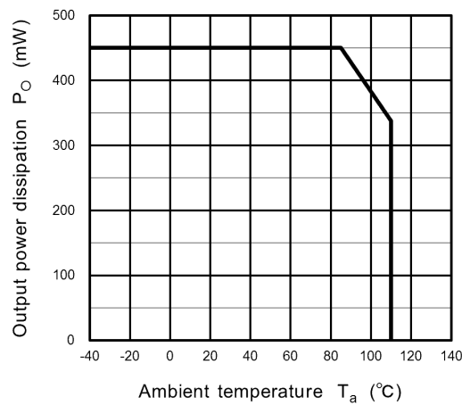
Fig. 13.2.3 P_O - T_a
