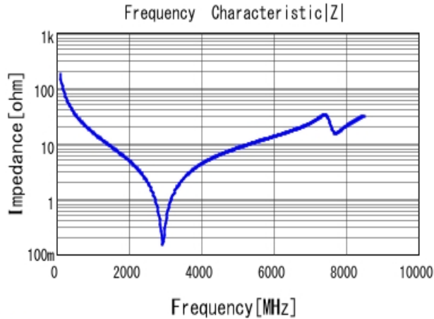
■ GCQ1555C1H9R0DB01 |Z| DC0V, 25degC
