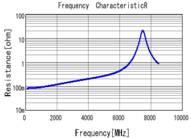
■ GCQ1555C1H9R0DB01 R DC0V, 25degC
