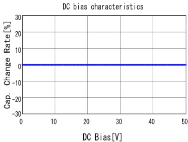
■ GCQ1555C1H9R0DB01 C-DC bias capchange, 25.0degC, AC1V
