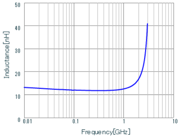
LQG18HN12NJ00 L.
