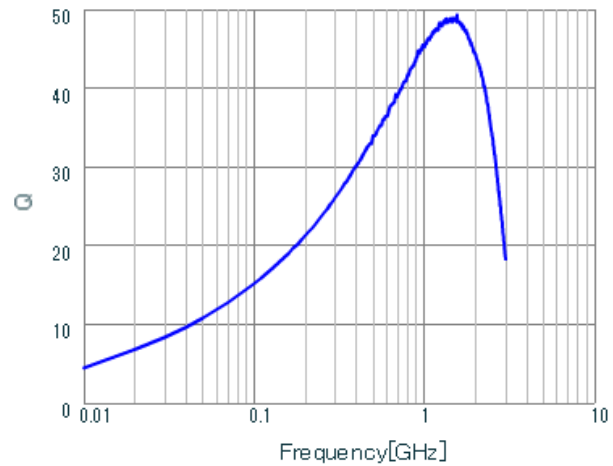
LQG18HN12NJ00 Q.
