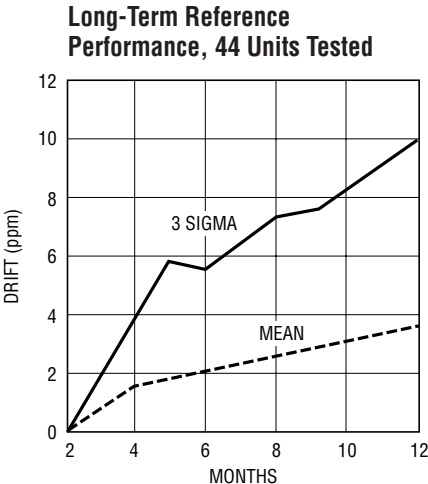
LM199 G10
