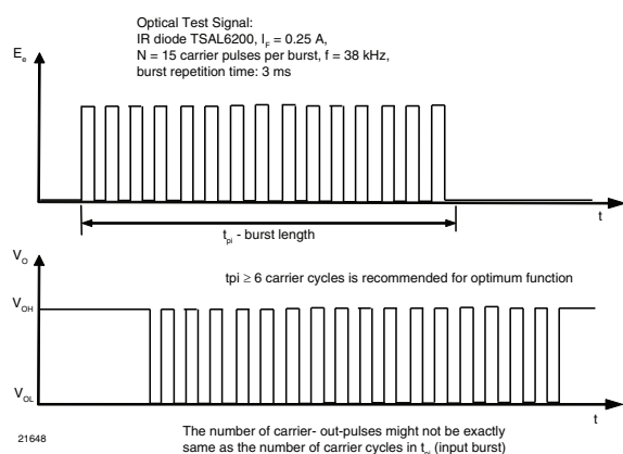
Fig. 1 - Output Function
