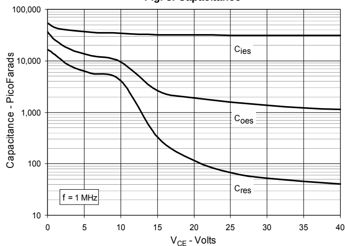
Fig. 8. Capacitance
