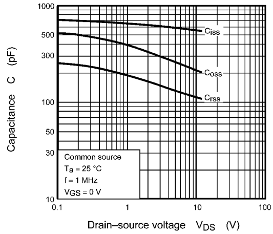
Fig. 7.10 C - V_{DS}
