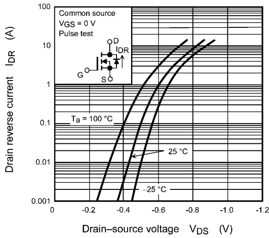
Fig. 7.9 I_{DR} - V_{DS}
