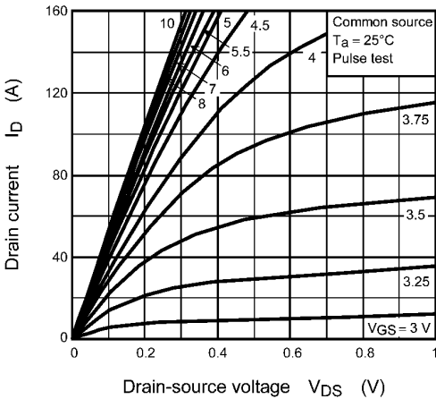
Fig. 8.2 I_D - V_{DS}
