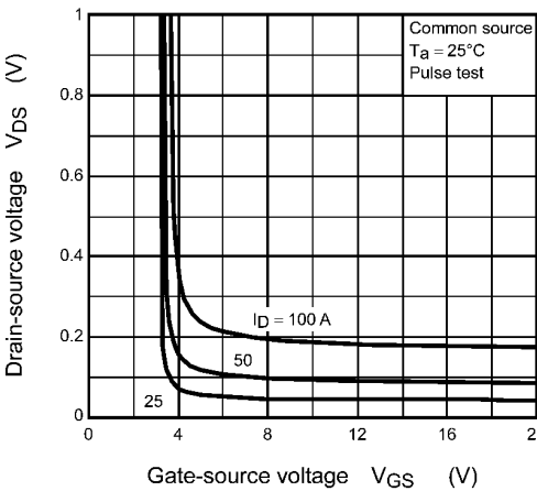
Fig. 8.4 V_{DS} - V_{GS}
