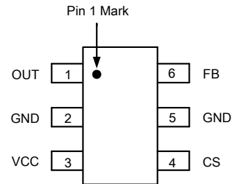
SOT26
