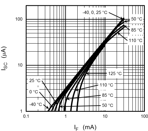
Fig. 12.6 I_{SC} - I_F
