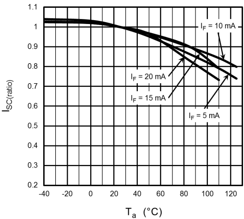
Fig. 12.10 I_{SC(ratio)} - T_a
