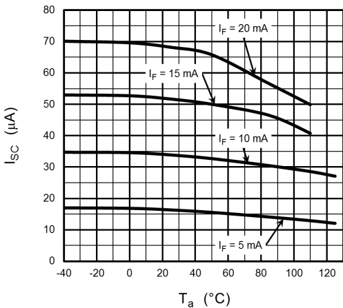
Fig. 12.9 I_{SC} - T_a
