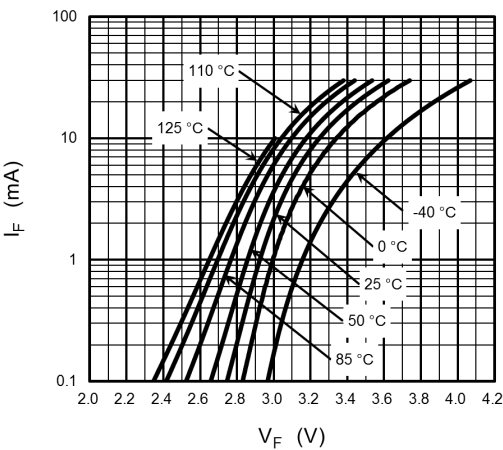
Fig. 12.2 I_F - V_F
