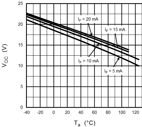
Fig. 12.7 V_{OC} - T_a
