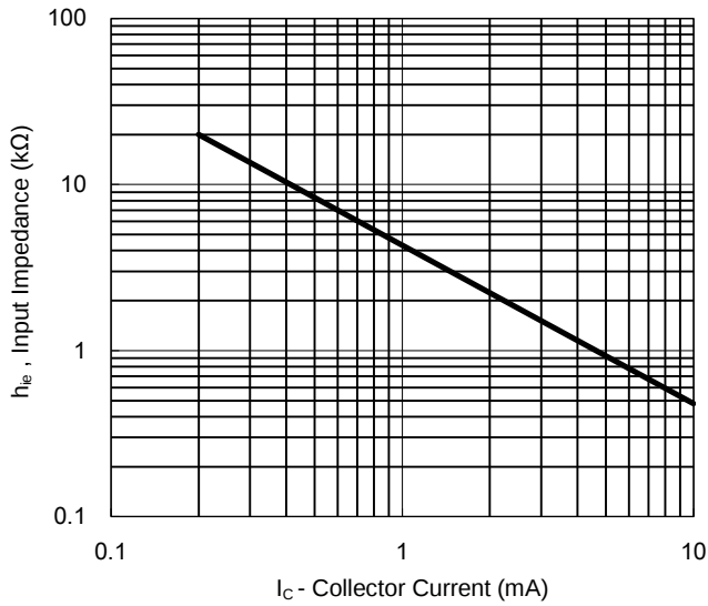
Fig.9 Input Impedance
