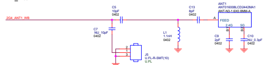
WL_BG/BT ANT1
