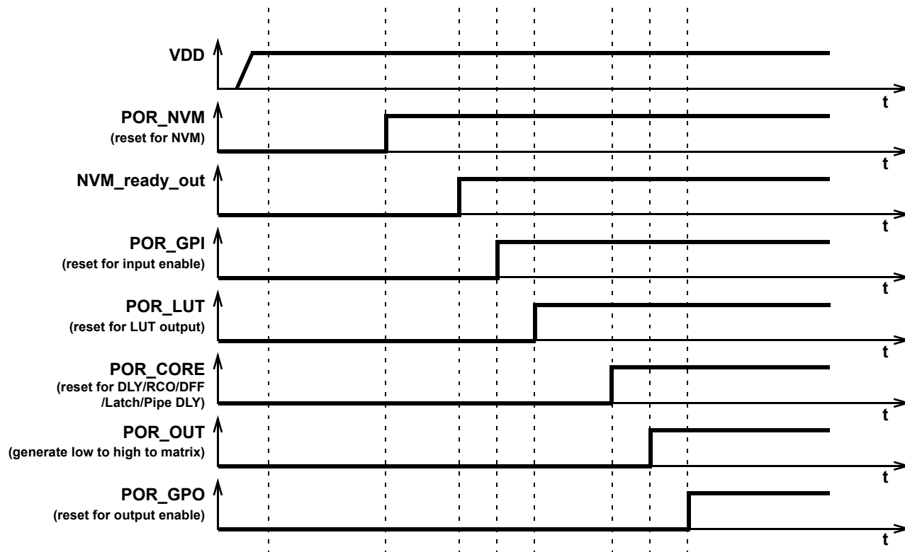
Figure 122. POR sequence
