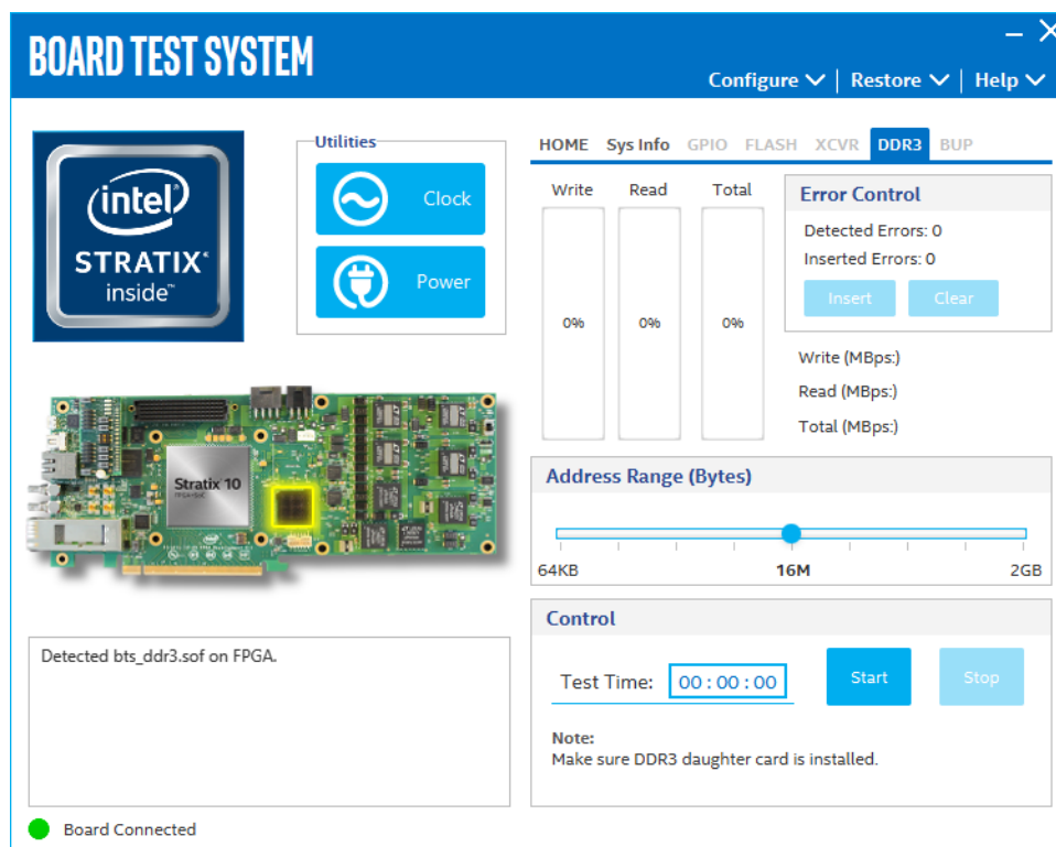
Figure 29. The DDR3 Tab
