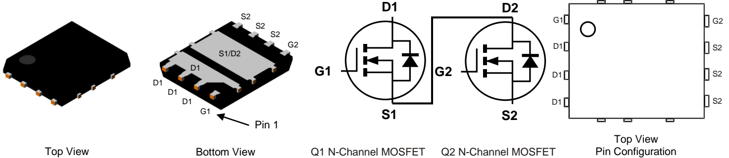
PowerDI5060-8 (Type S)
