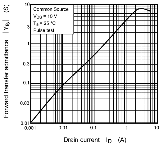
Fig. 8.7 |Y_{fs}| - I_D
