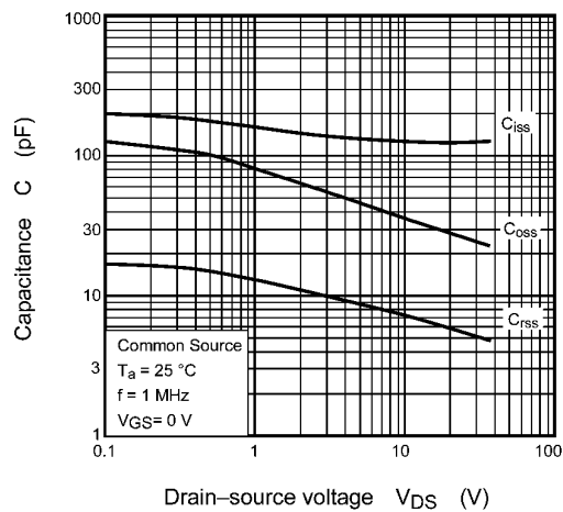
Fig. 8.9 C - V_{DS}
