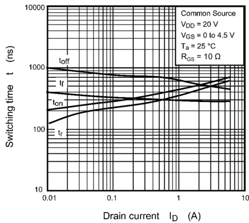
Fig. 8.10 t - I_D
