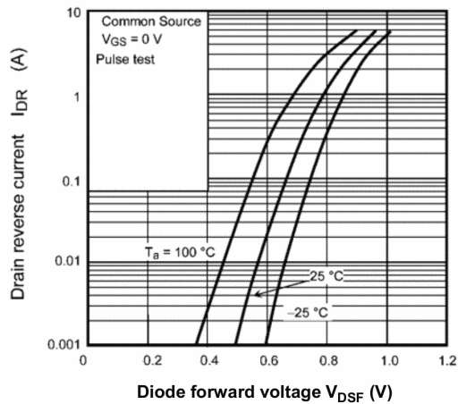
Fig. 8.8 I_{DR} - V_{DSF}
