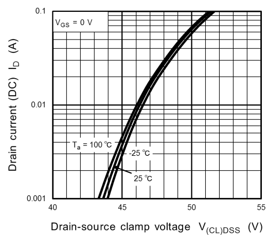
Fig. 8.14 I_D - V_{(CL)DSS}
