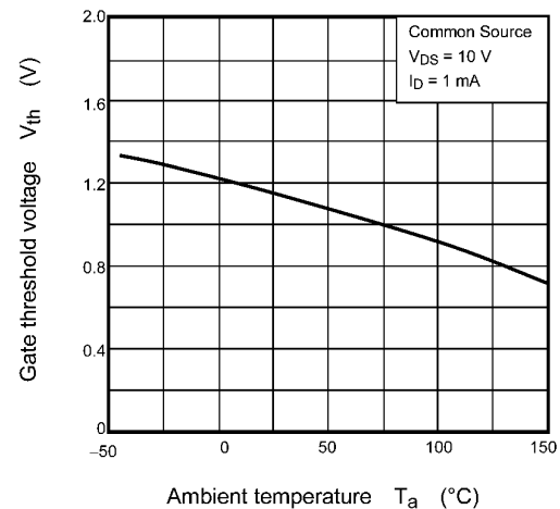
Fig. 8.6 V_{th} - T_a
