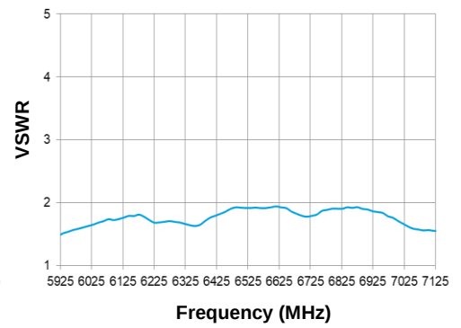
6 / 7 GHz VSWR
