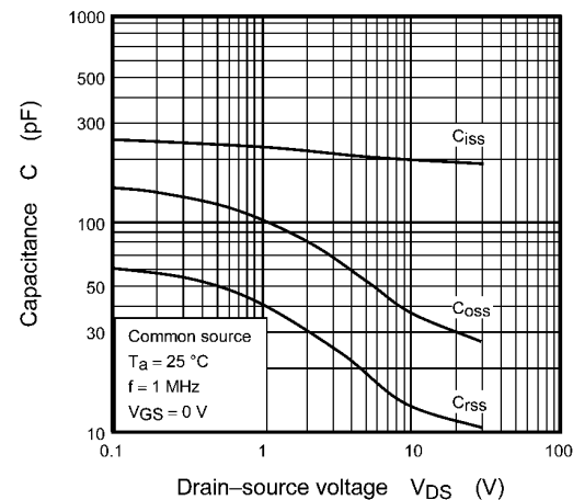
Fig. 9.10 C - V_{DS}
