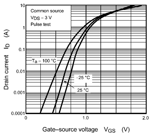
Fig. 9.2 I_D - V_{GS}
