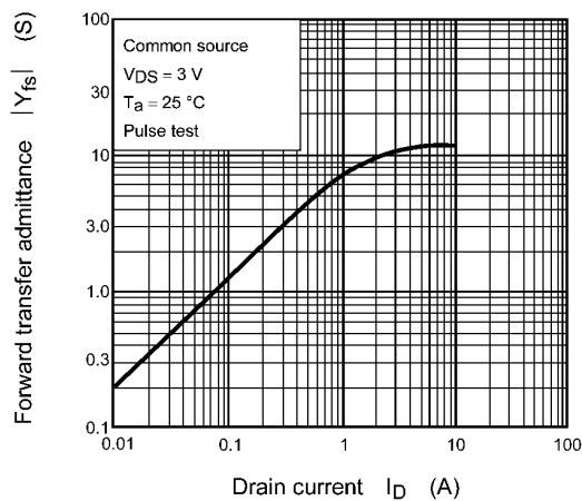
Fig. 9.8 |Y_{fs}| - I_D
