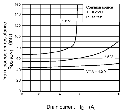
Fig. 9.5 R_{DS(ON)} - I_D
