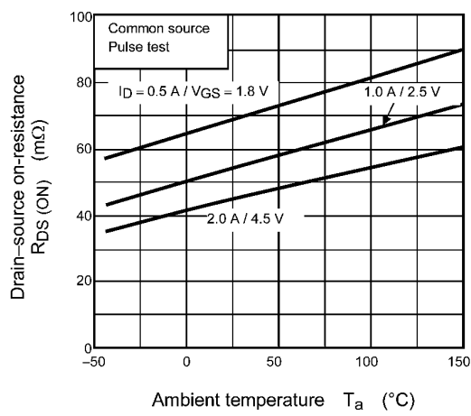
Fig. 9.6 R_{DS(ON)} - T_a
