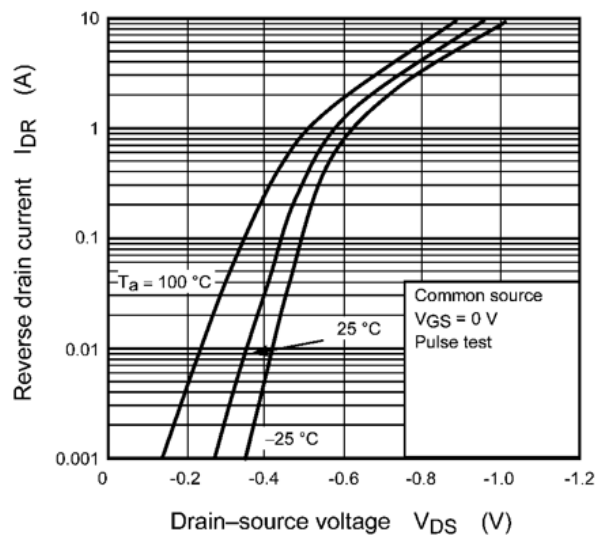
Fig. 9.9 I_{DR} - V_{DS}
