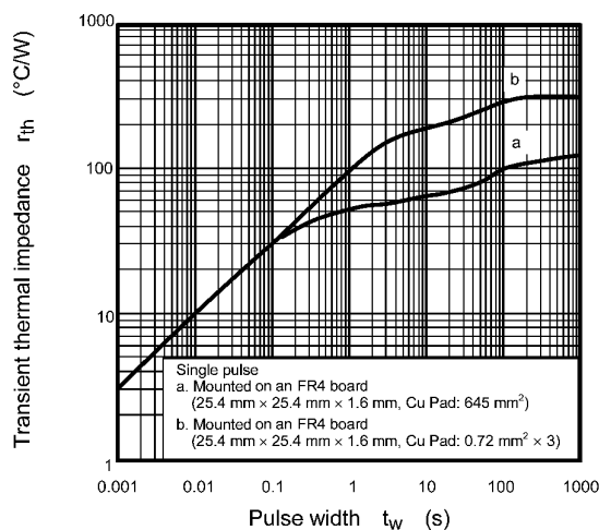
Fig. 9.13 r_{th} - t_w
