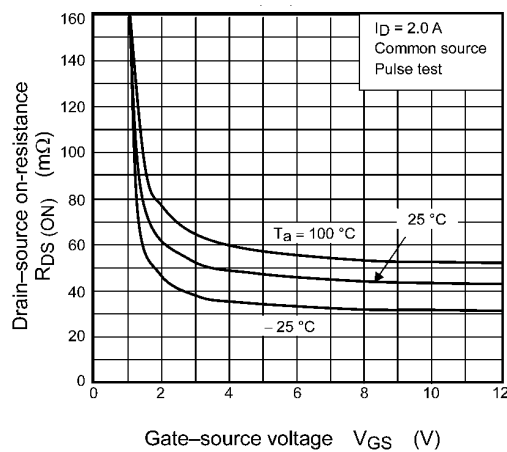
Fig. 9.4 R_{DS(ON)} - V_{GS}
