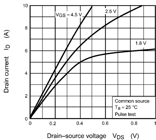
Fig. 9.1 I_D - V_{DS}
