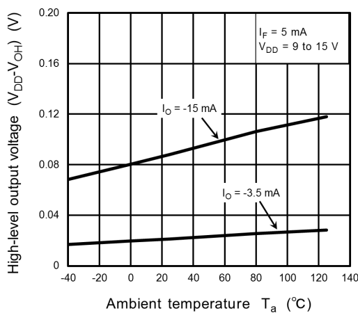
Fig. 12.2.6 (V_{DD} - V_{OH}) - T_a
