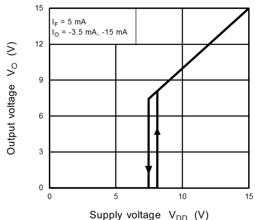
Fig. 12.2.11 V_O - V_{DD}
