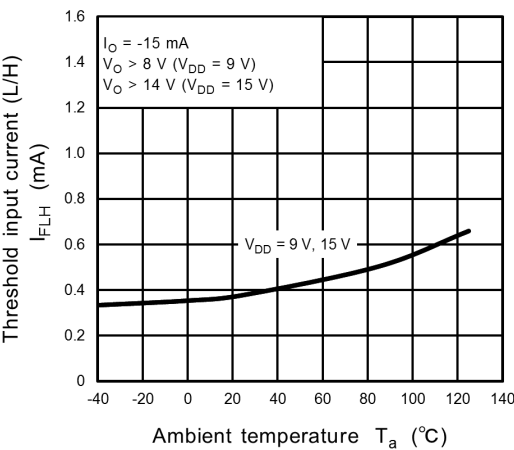
Fig. 12.2.2 I_{FLH} - T_a
