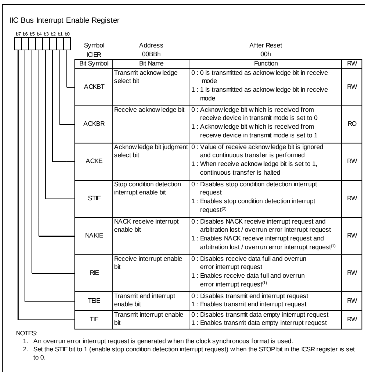
Figure 16.27 ICIER Register
