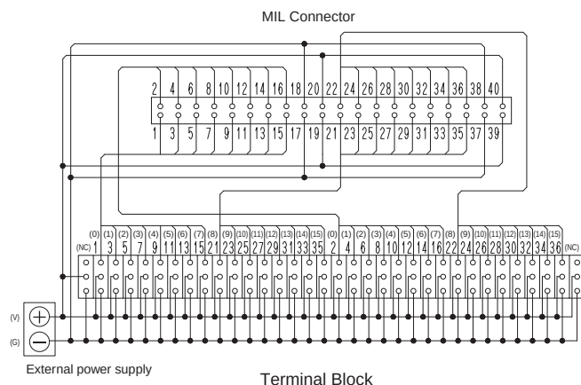
XW2R-P32GD-C3-COM
