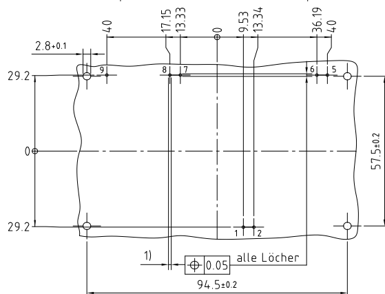
Leiterplatten-Lochbild / PCB drillhole pattern
