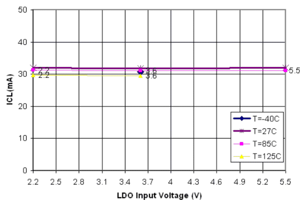
Figure 28. LDO MINI Short-Circuit Current Limit vs V I
