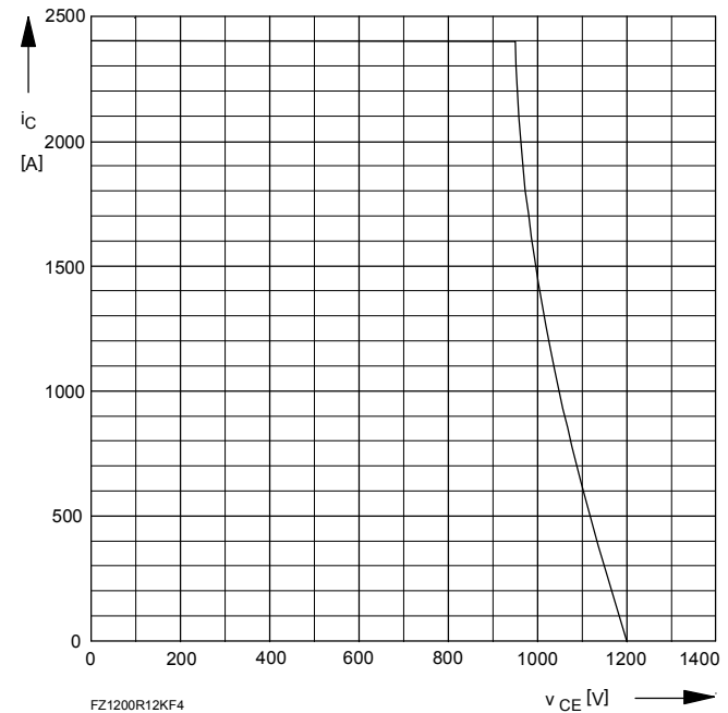
Bild/Fig. 4 Rückwärts-Arbeitsbereich Reverse biased safe operating area t_{vj} = 125\text{ °C} , v_{LE} = v_{LR} = 15V , R_G = 0,82\Omega
