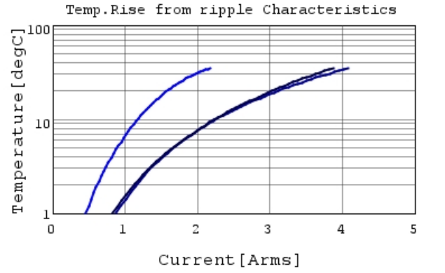
GJ821BR71H105KA12 Temp.rise — 100kHz —
