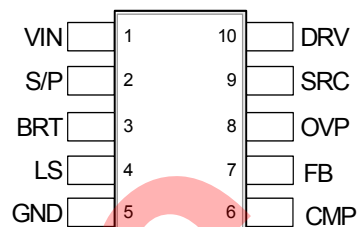
DU PACKAGE (Top View)
