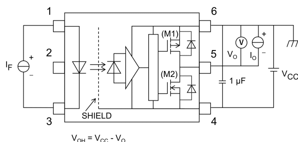
Fig. 13.1.3 V_{OH} Test Circuit
