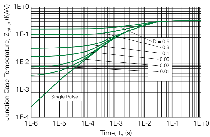
Fig. 25. Thermal Impedance
