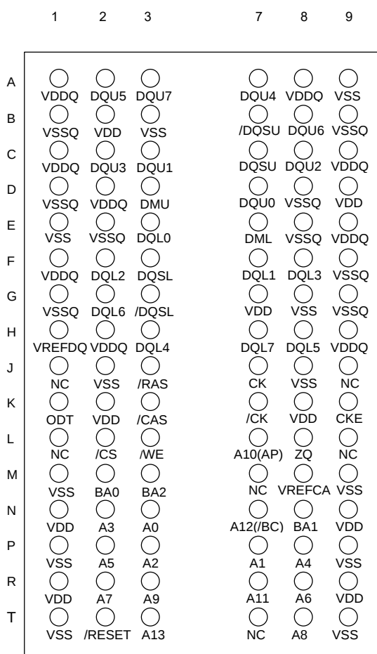
96-ball FBGA
