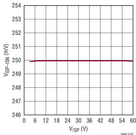
V ISP-ISO vs V ISP
