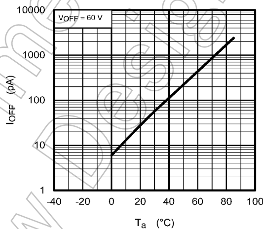
Fig. 13.1.10 I_{OFF} - T_a
