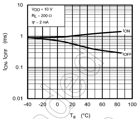
Fig. 13.1.8 t_{ON} , t_{OFF} - T_a
