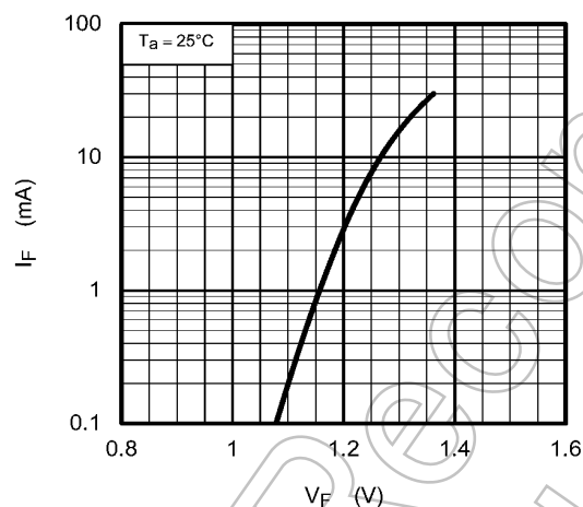
Fig. 13.1.3 I_F - V_F
