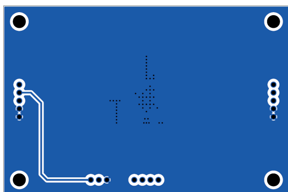
Layer 3 (GND)
