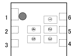
USP-6C
