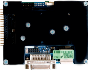
pITX-SP incl. mounted Heatspreader
