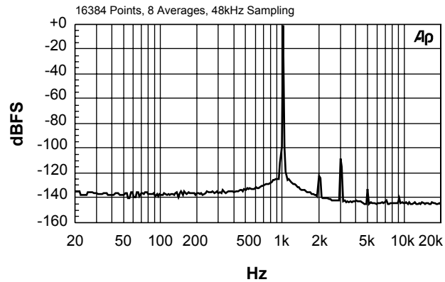
0dB FFT
