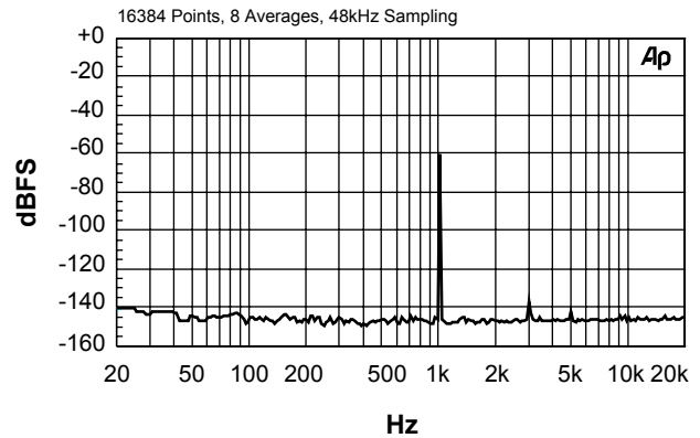
-60dB FFT
