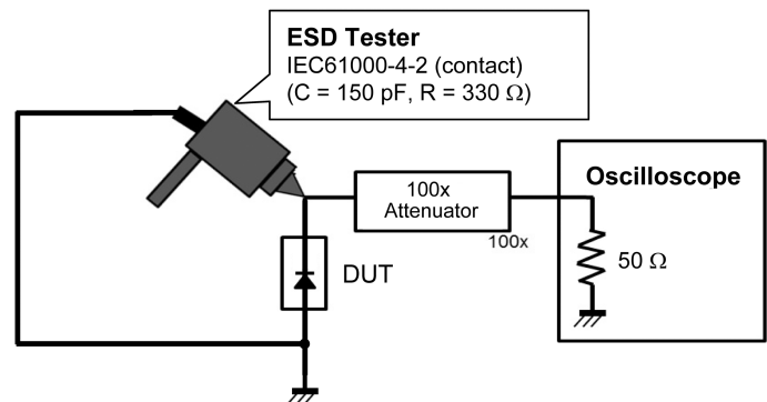
Fig. 6.1.5 IEC61000-4-2 (Contact)
