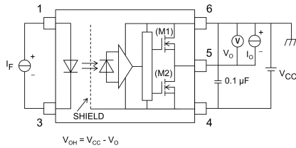
Fig. 12.1.3 V_{OH} Test Circuit
