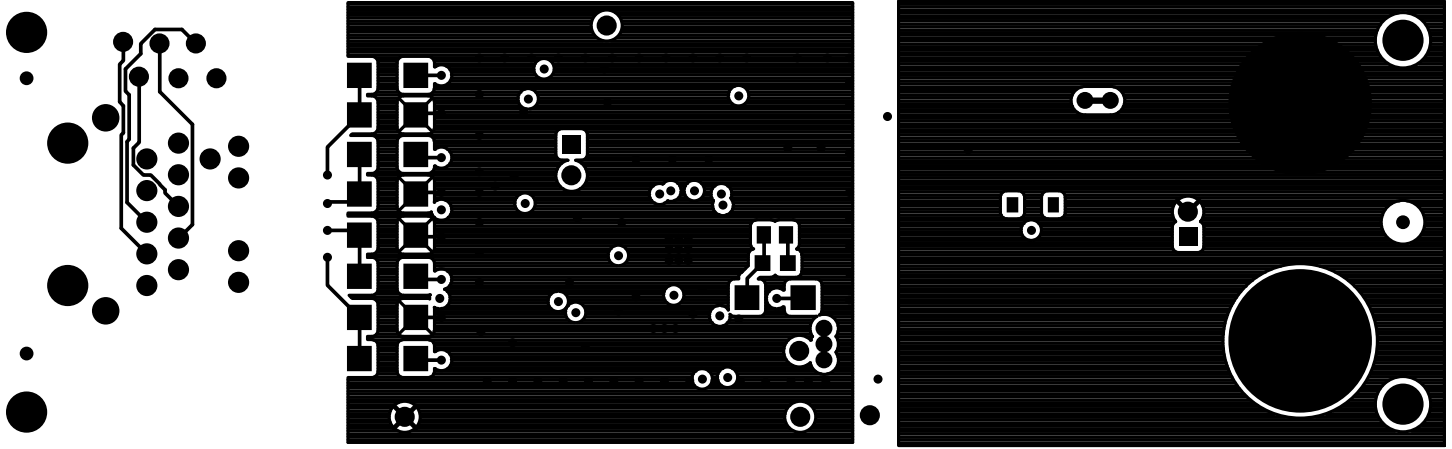
Figure 17.5. Bottom Layer
