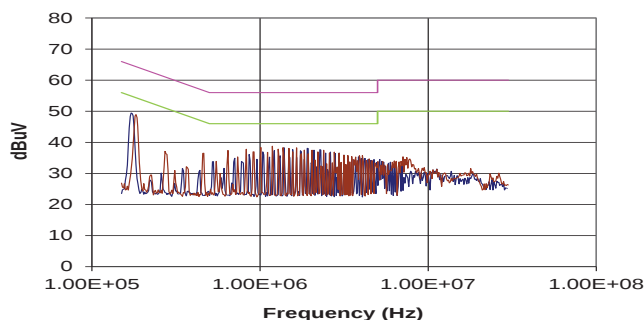
MGJ1D121505MPC
