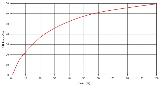
MGJ1D151505MPC
