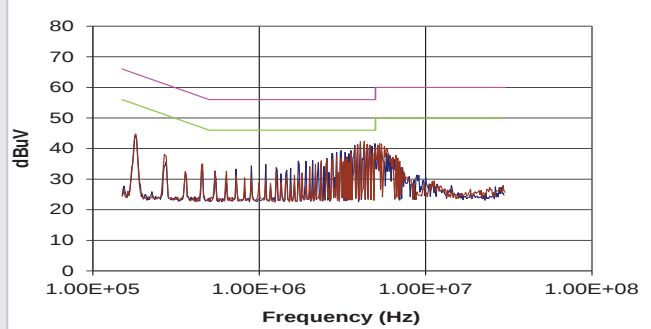
MGJ1D121905MPC
