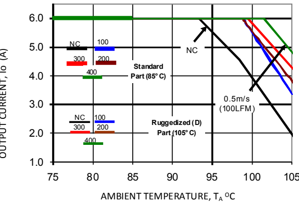
Vo=5.0V
