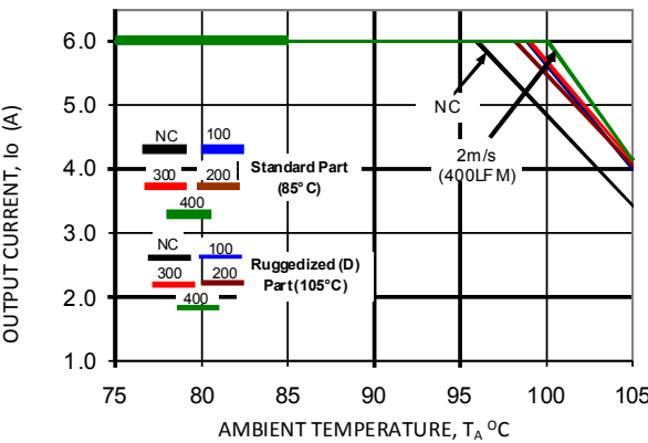
Vo=1.2V
