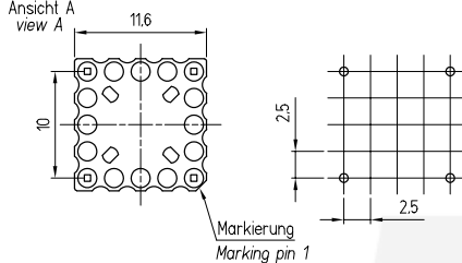
Ansicht A view A
