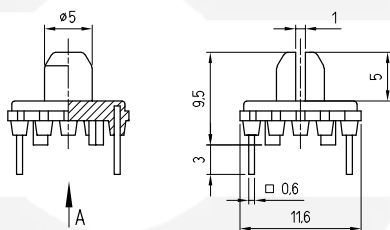
Ansicht A view A
