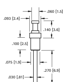
Feed-Thru
