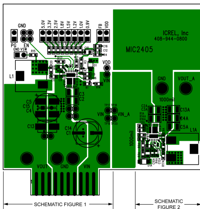
Top Layer
