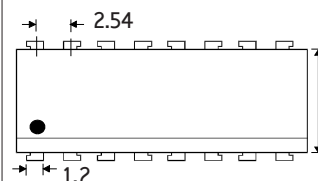
TLP620-4
