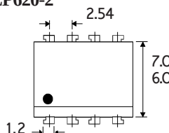
TLP620-2
