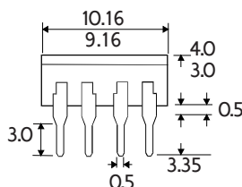
TLP620-4
